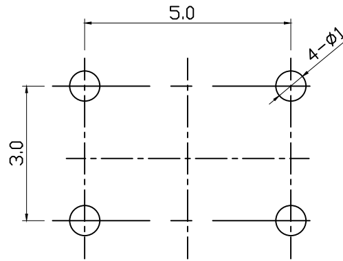
P.C.B Holes Diagram
