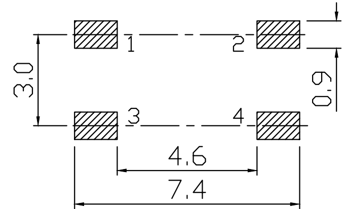
P.C.B Holes diagram
