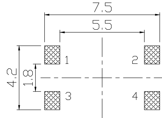
P.C.B Holes diagram
