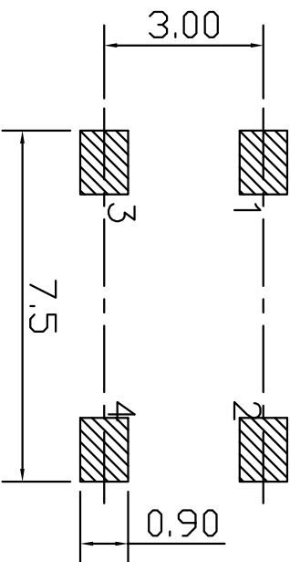
P.C.B Holes diagram
