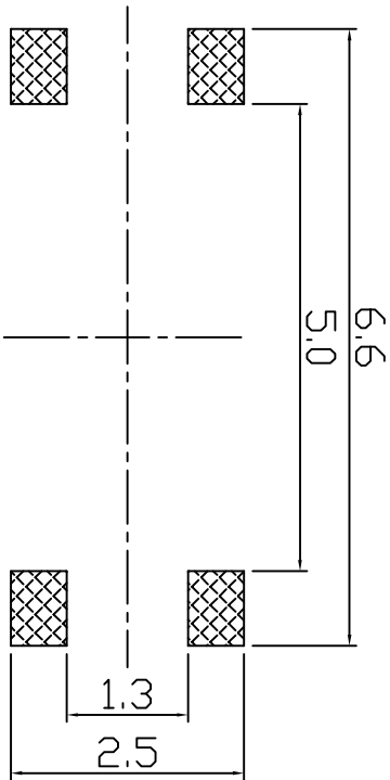
P.C.B. LAYOUT
